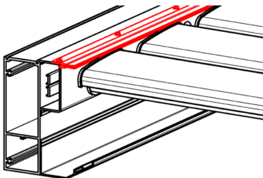
Petite broche d'étanchéité côté moteur
