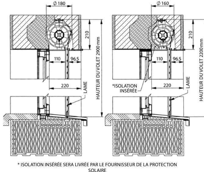
INSTALLATION DE CHÂSSIS DE FENÊTRE POUR LES VOILETS ROULANTS, 220MM DE LA PARTIE EXTÉRIEURE DU REVÊTEMENT DE LINTEAU
