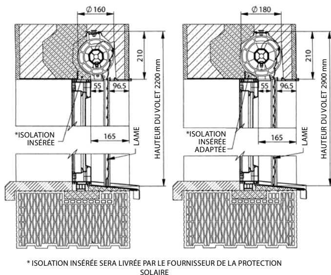
INSTALLATION DE CHÂSSIS DE FENÊTRE POUR LES VOILETS ROULANTS, 165MM DE LA PARTIE EXTÉRIEURE DU REVÊTEMENT DE LINTEAU
