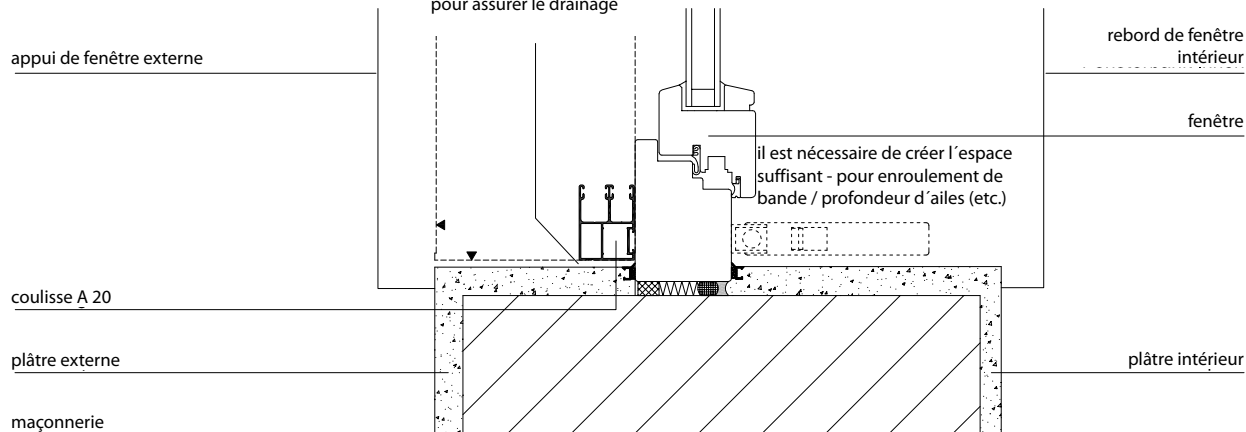
Détail de connexion - vue du côté (partie basse)
