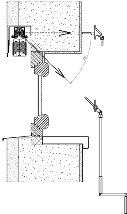
Montage du store dans la niche sur un profil s'élargissant (plafond/mur)
