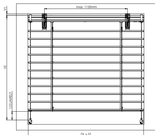
Guidage par câble - verticale
