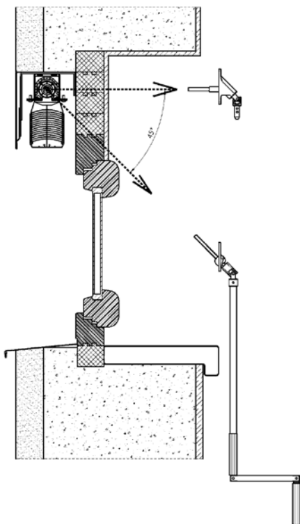
Montage du store dans la niche sur un profil s'élargissant (plafond/mur)
