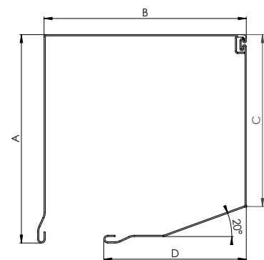
Box plié, 20°
