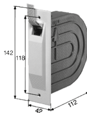
Bobineur de bande encastré PR0133 6-001913-XXXX Version de couleur: blanc, brun
