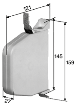
Bobineur de bande PR0131 6-001908-XXXX Version de couleur: blanc, brun
