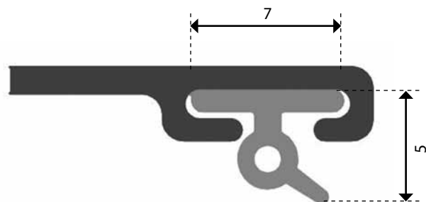
Insert d'étanchéité stabilisateur en PVC PR0430 6-001796-0000
