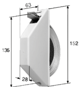
Bobineur de bande semi-encastré PR0286 6-003640-XXXX Version de couleur: blanc, brun
