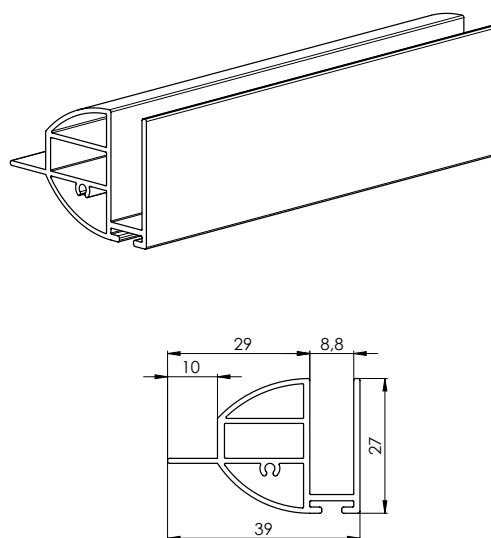
Cooulisse spéciale, de terminaison (6-012001)
