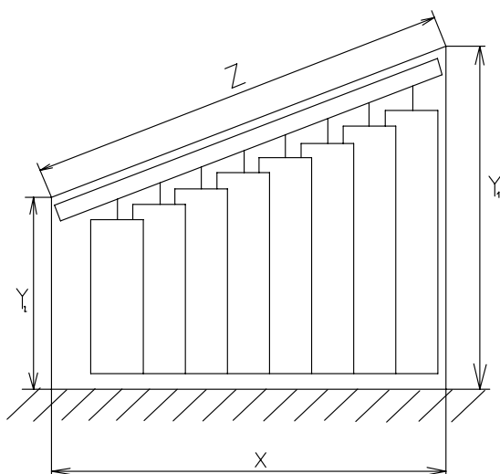
store incliné
