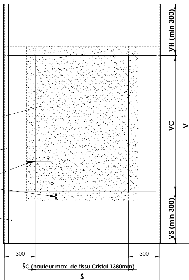
VERSION DE TISSU CIRISTAL POUR LES PRODUITS SCREEN ZIP ET SCREEN ZIP ECONOMY
