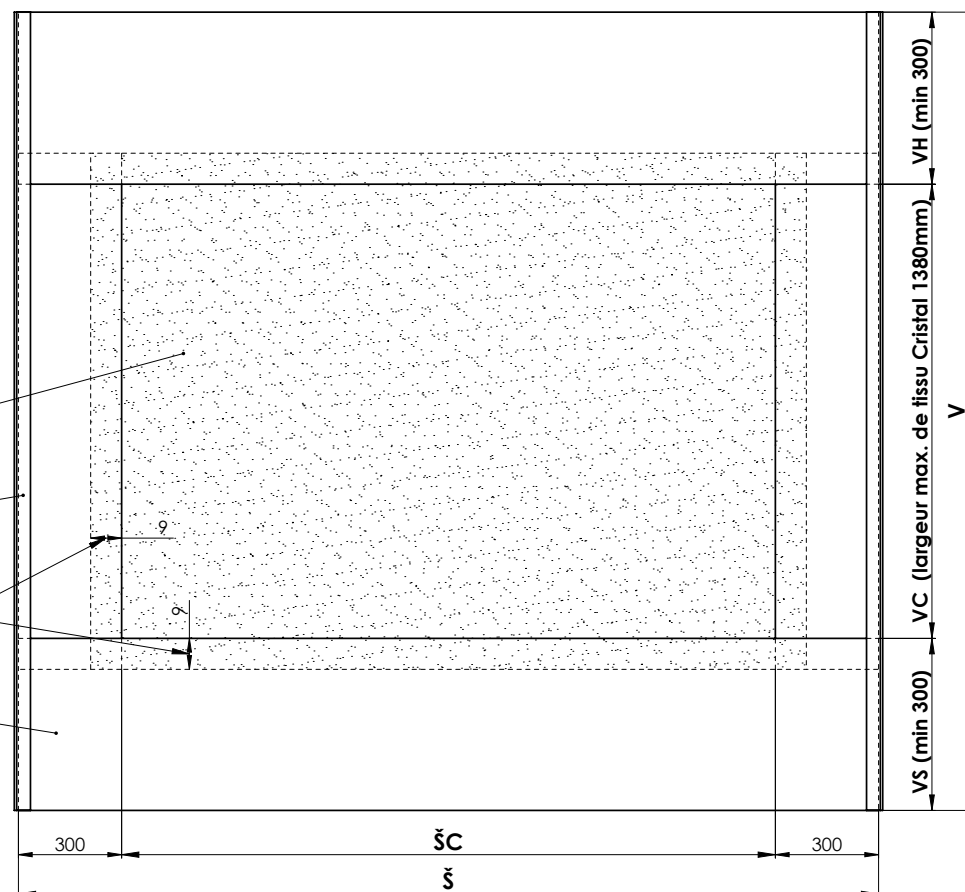
VERSION HORIZONTALE DE TISSU CRISTAL POUR LES PRODUITS SCREEN ZIP ET SCREEN ZIP ECONOMY
