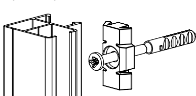
Équerres pour coulisses 829, 839, 855, 865
