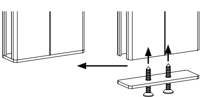
Fin de course sur la coulisse auxiliaire
