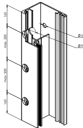
A840-1c la perçage frontal
