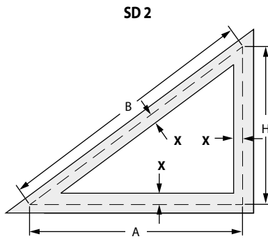
Dimensions pour la commande* = A et H
