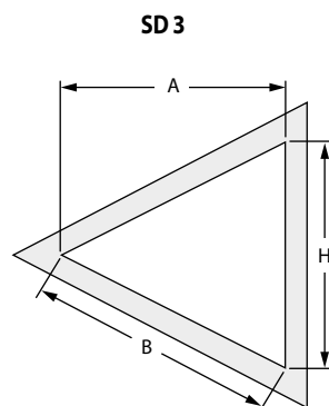
Dimensions pour la commande* = A, BK, B2K et H
