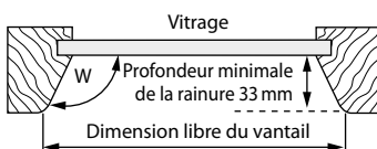
L'aile est toujours avec une rainure oblique
