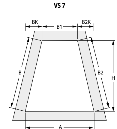
Dimensions pour la commande* = A, B1, Bk, B2k, et H
