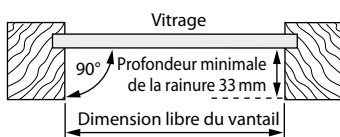
Aile avec une rainure droite
