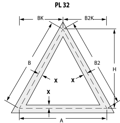
Dimensions pour la commande* = A, BK, B2K et H
