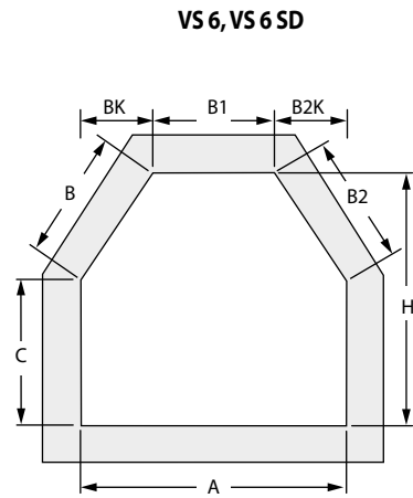
Dimensions pour la commande* = A, B1, Bk, B2k, H et C
