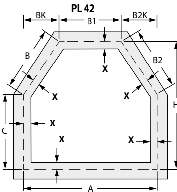
Dimensions pour la commande* = A, B1, BK, B2K, H et C
