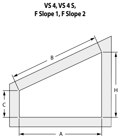
Dimensions pour la commande* = A, H et C
