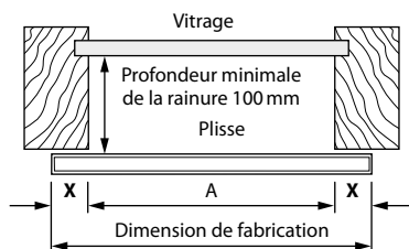
Dimensions pour la commande* = A, B1, BK, B2K, H et C
