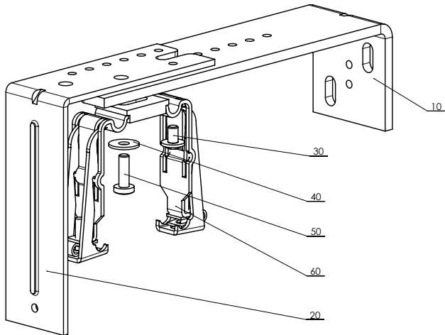
Support réglable - mécanique 206 – 268 mm P 010/36 (2-01794-0000)
