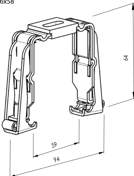
Etrier du boîtier - Fe Click P 002/32 (7-201862-0000) 56x58
