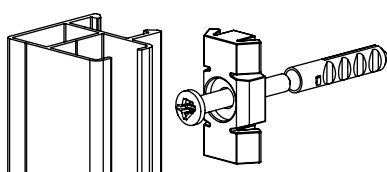
Équerres pour coulisses 829, 839, 855, 865
