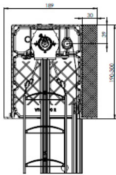
Coupe de store autoportant encastred Viva (Prepare pour le polystyrene de cote frontal + styrodur 30 de cote arriere)
