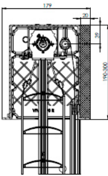
Coupe de store autoportant encastred Viva (Prepare pour le polystyrene de cote frontal + styrodur 20 de cote arriere)
