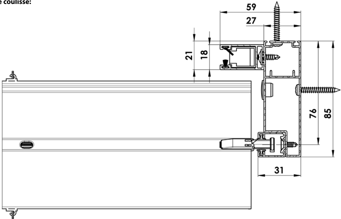
Coupe coulisse:
