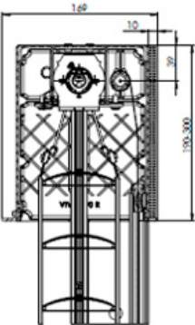
Coupe de store autoportant encastred Viva (Prepare pour le polystyrene de cote frontal + Alutermo quatre 10 de cote arriere)
