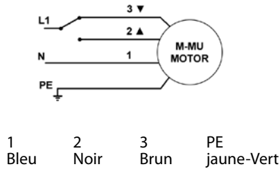
Schéma de branchement de moteur
