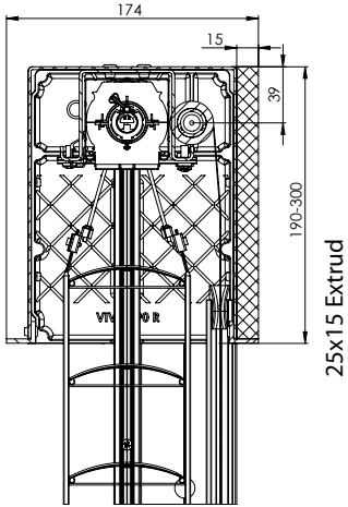
Coupe de store autoportant Viva (prepare pour le polystyrene dans une partie frontale+ polystyrene a l'arriere. Isolation thermique derriere le box seulement 15 mm sans tenir compte du decalage du box !
