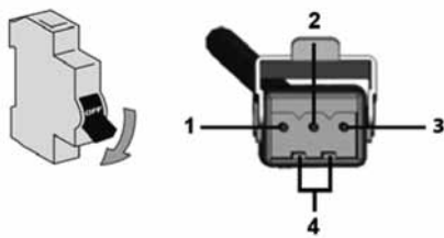
Schéma de branchement de moteur RTS / IO
