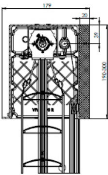
Coupe de store autoportant encastré Viva (Préparé pour le polystyrène de côté frontal + styrodur 20 de côté arriere)
