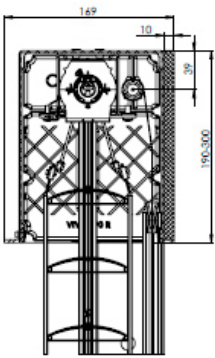
Coupe de store autoportant encastré Viva (Préparé pour le polystyrène de côté frontal + styrodur 10 de côté arriere)
